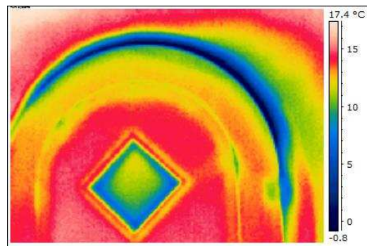
Beispiel: Undichte Hauseingangstür
