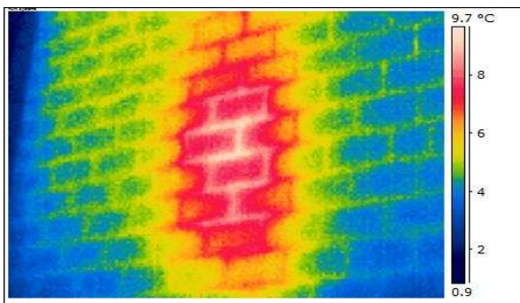
Beispiel: Heizkörper hinter der Wand
