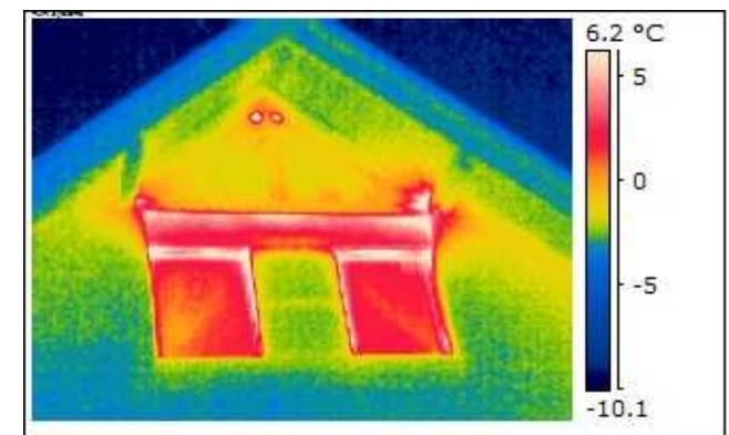
Beispiel: Ungedämmter Rollladenkasten
