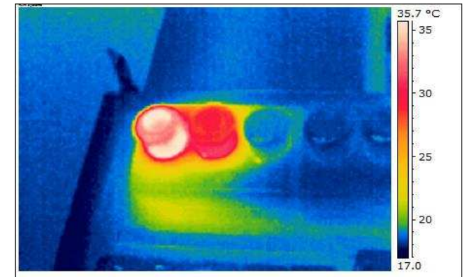
Beispiel: Überhitzte Sicherung in Unterverteilung
